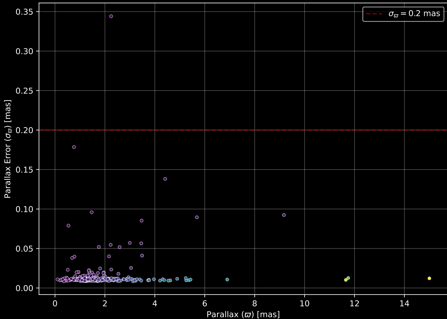
GALAH DR4 Field: [559] Parallax Quality (n= 300)
