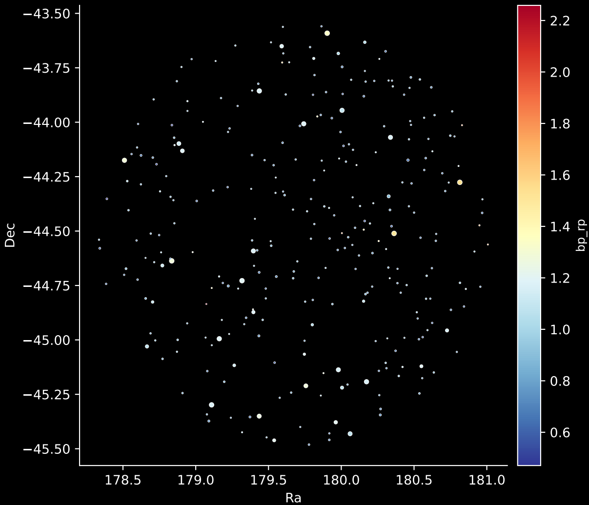
GALAH DR4 Field: [559] Stars: 300
