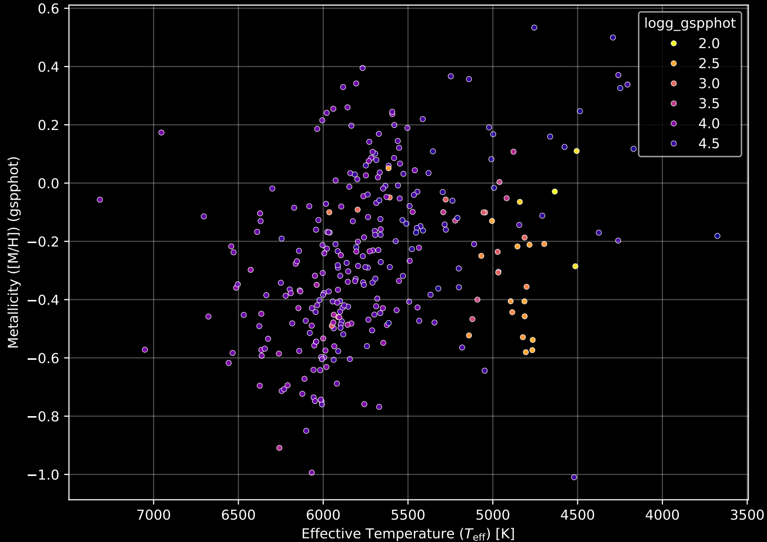
GALAH DR4 Field: [559] Stellar Population Parameters (n= 300)
