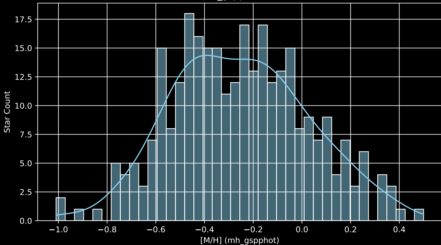
GALAH DR4 Field: [559] [M/H] (mh_gspphot) (n= 299)
